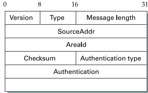
Figure 4.19 OSPF header format.
